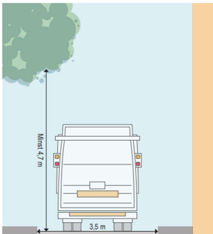
Bild 5. Exempel på transportvägs bredd och fria höjd, bild från Handbok för avfallsutrymmen, Avfall Sverige
