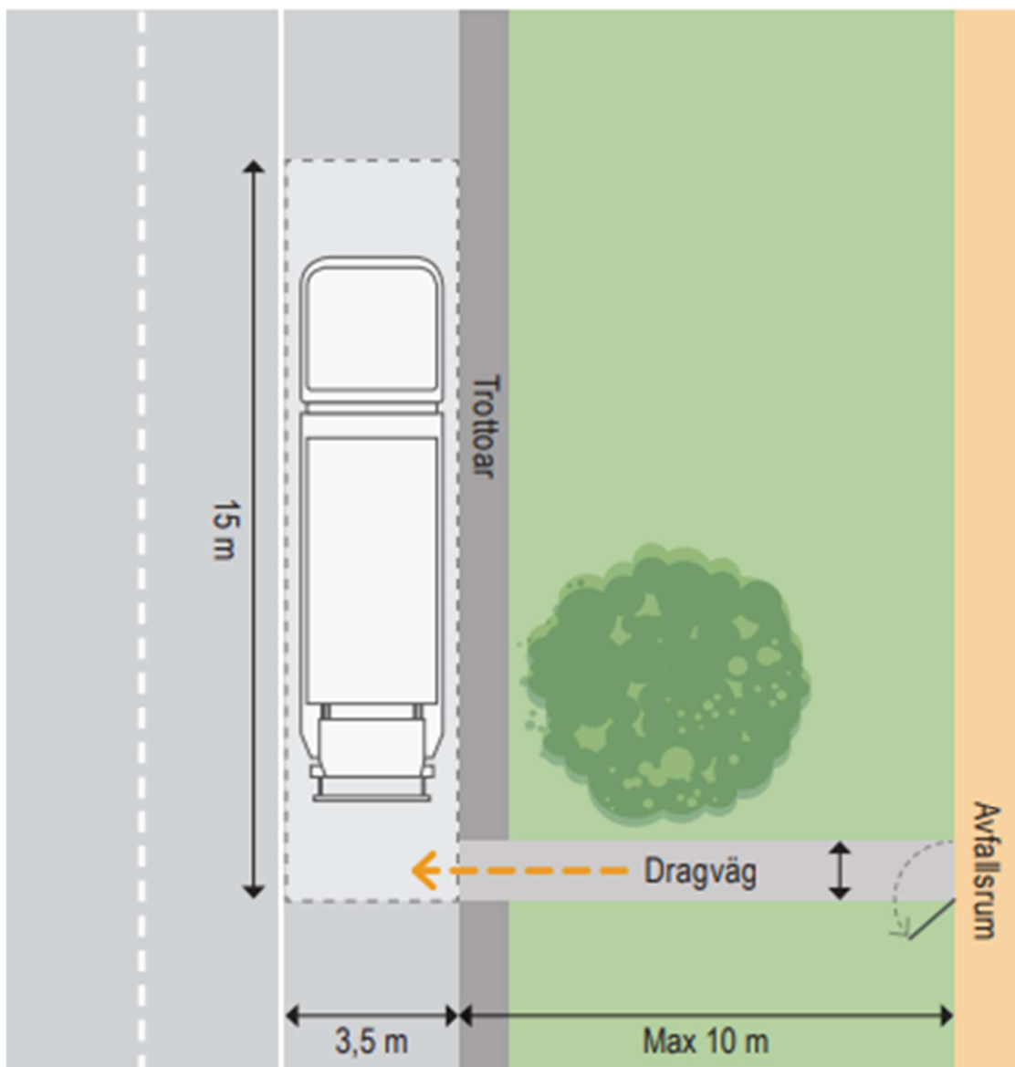
Bild 3. Dragväg, bild från Handbok för avfallsutrymmen, Avfall Sverige
