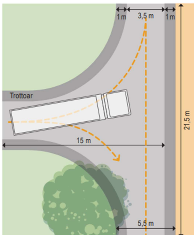
Bild 5. Exempel på transportvägs bredd och fria höjd, bild från Handbok för avfallsutrymmen, Avfall Sverige
