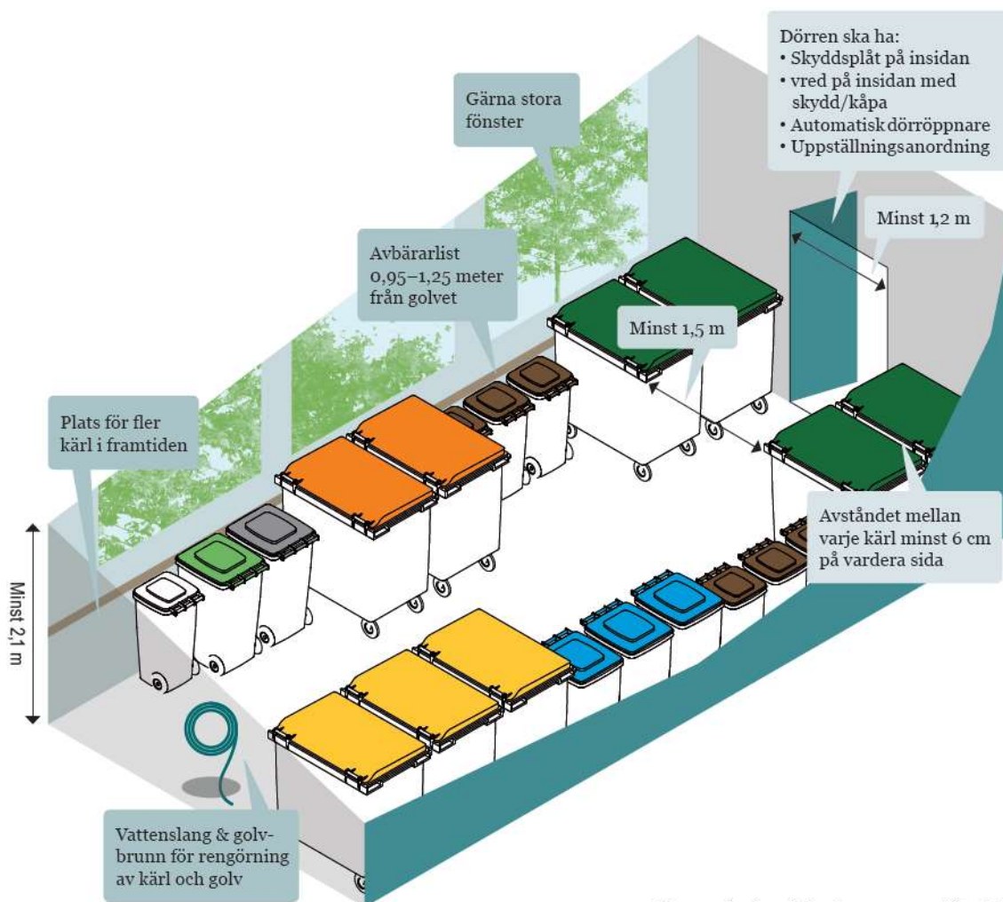
Bild 1. Exempel på avfallsutrymme i flerbostadshus, bild från Handbok för avfallsutrymmen, Avfall Sverige
